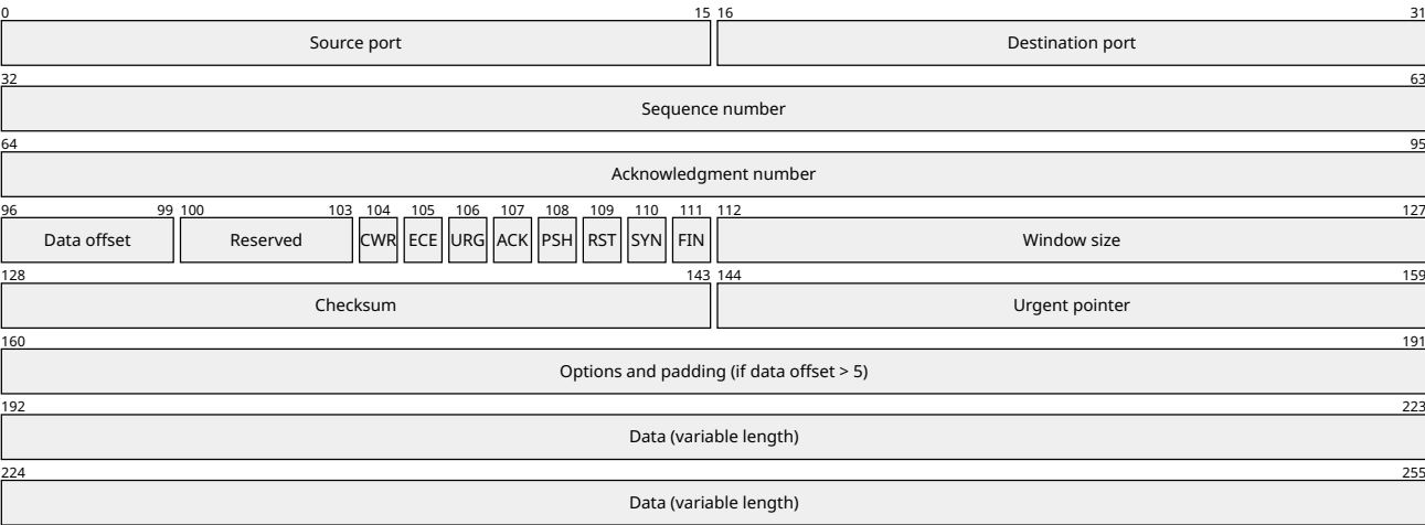
TCP header
